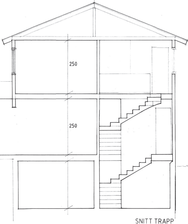
SNITT TRAPP
