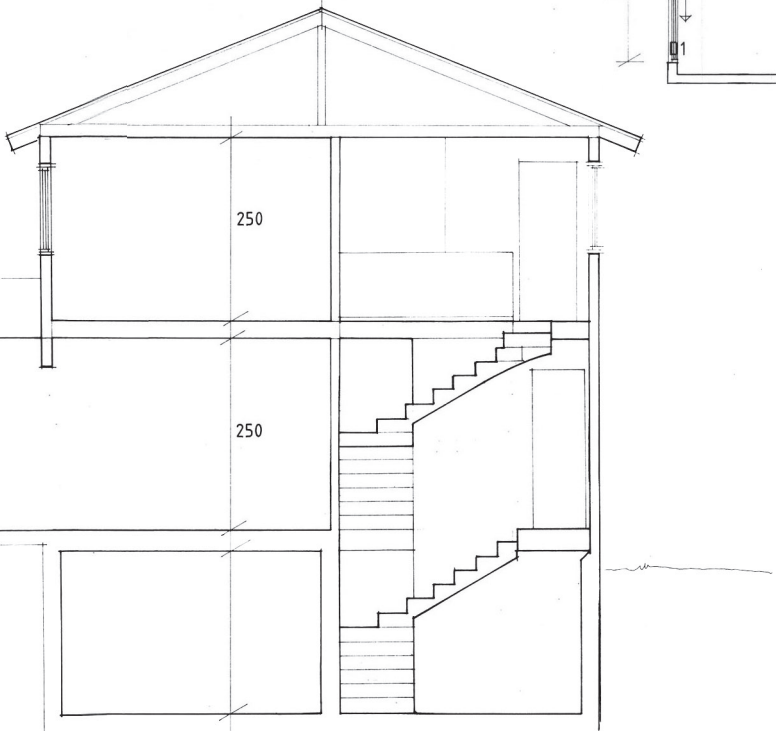
SNITT TRAPP
